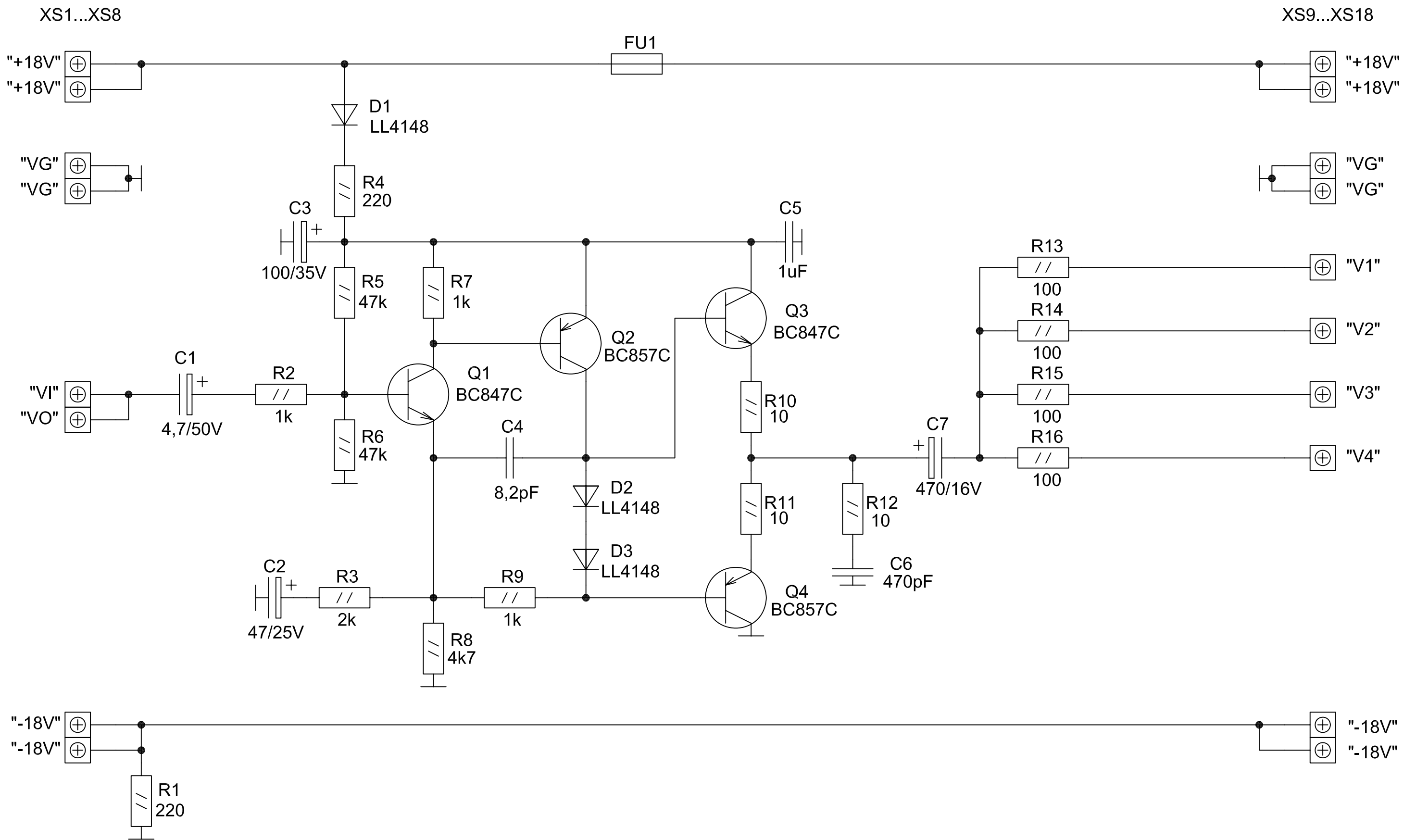
Разветвитель видеосигнала PVC-4 Схема электрическая принципиальная
