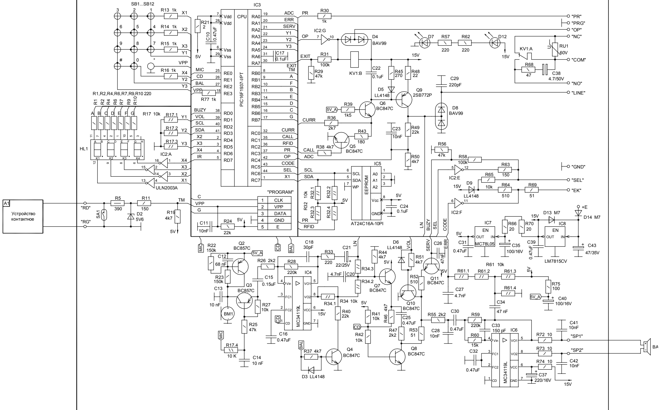
Блок вызова домофона БВД-SM101T
