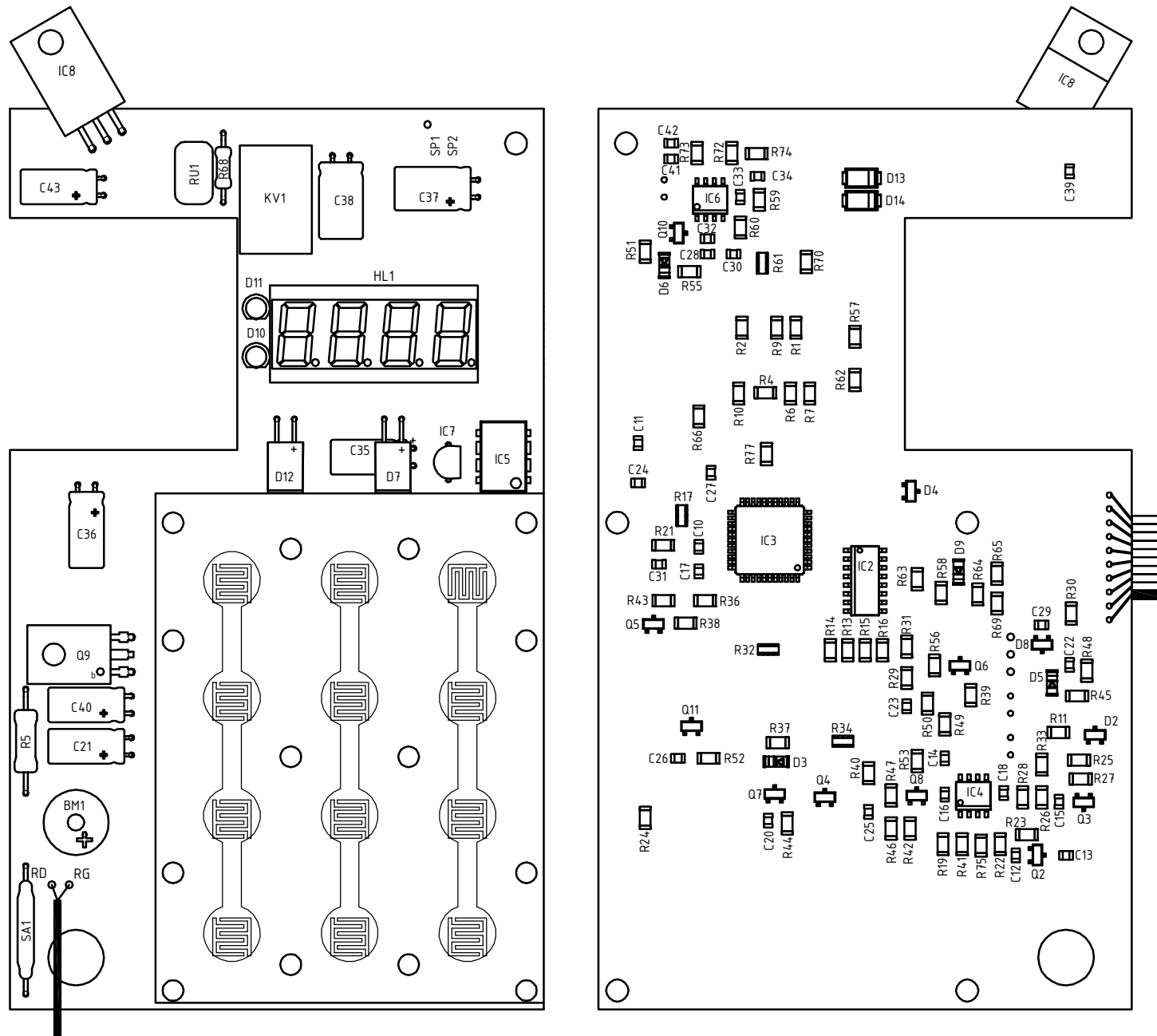
Плата БВД-СМ101Т Сборочный чертёж
