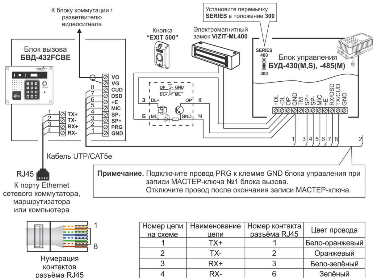
Рисунок 8.2 – Схема соединений блока вызова БВД-432FCBE с блоком управления БУД-430(М,S), -485(М), электромагнитным замком VIZIT-ML400 и кнопкой EXIT 500
