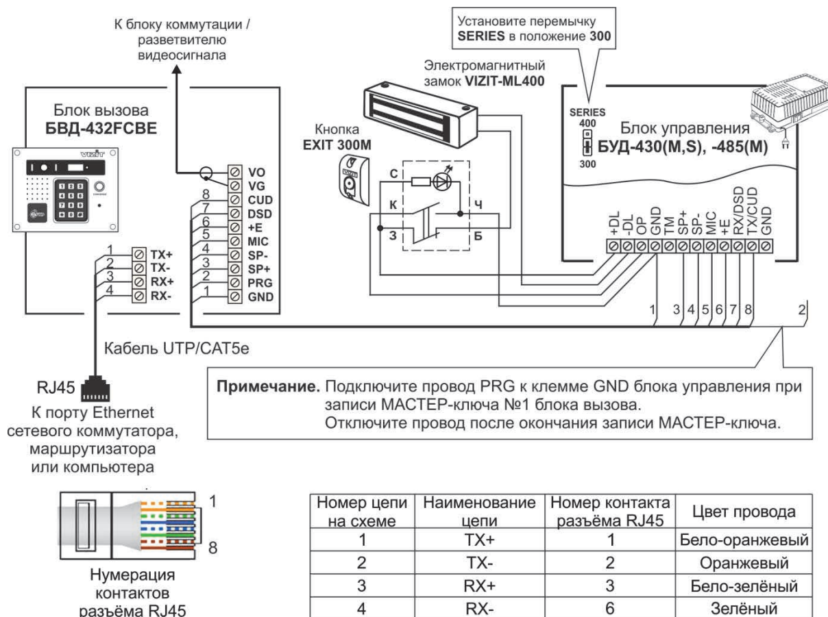
Рисунок 8.1 – Схема соединений блока вызова БВД-432FCBE с блоком управления БУД-430(М,S), -485(М), электромагнитным замком VIZIT-ML400 и кнопкой EXIT 300M
