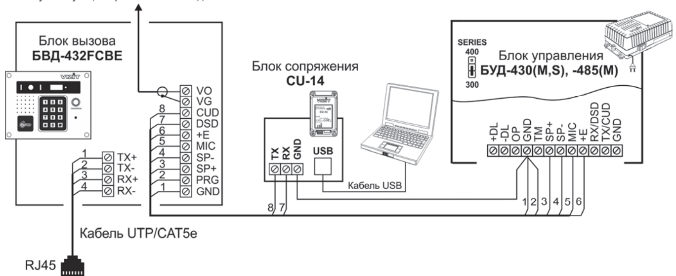
Рисунок 15.1 - Схема соединений блока вызова с блоками управления БУД-430(S, М), -485(М) и блоком сопряжения CU-14
