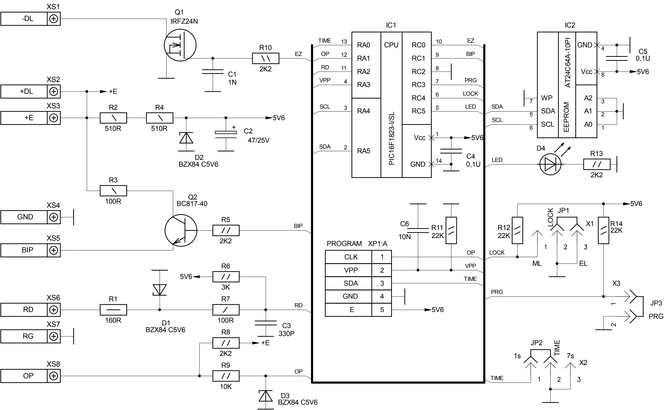
Контроллер VIZIT-KTM600R Схема электрическая принципиальная
