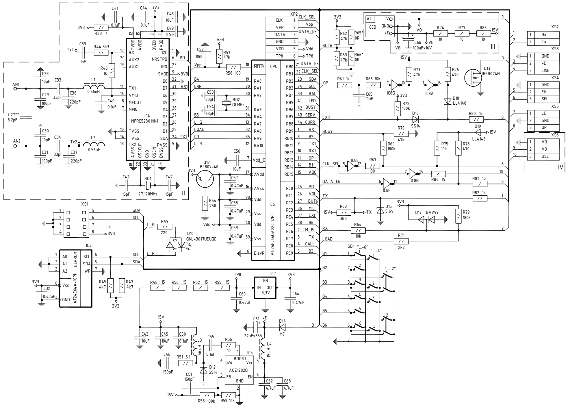
Блок вызова БВД-306х Схема электрическая принципиальная
