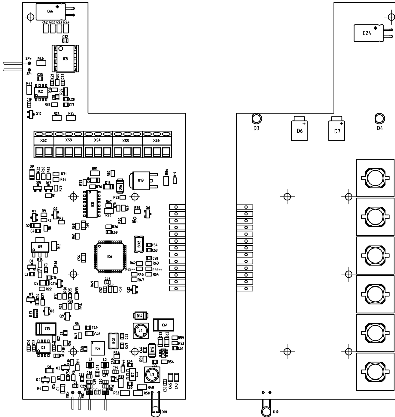
Плата БВД-306ФСР-6 Сборный чертеж
