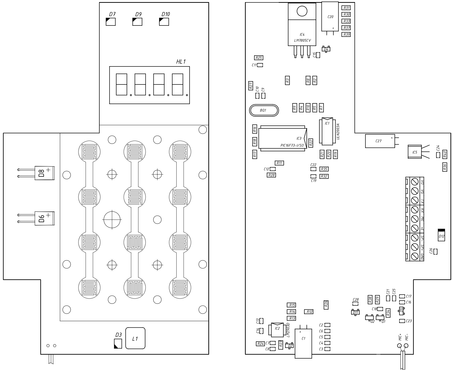
Плата БВД-343RCP Сборочный чертёж
