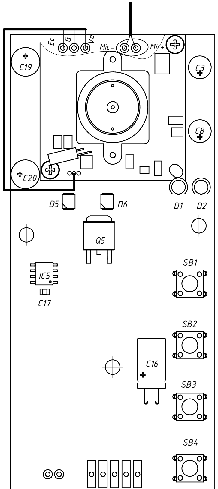
Плата БВД-405СР-2, БВД-405СР-4 Сборочный чертеж
