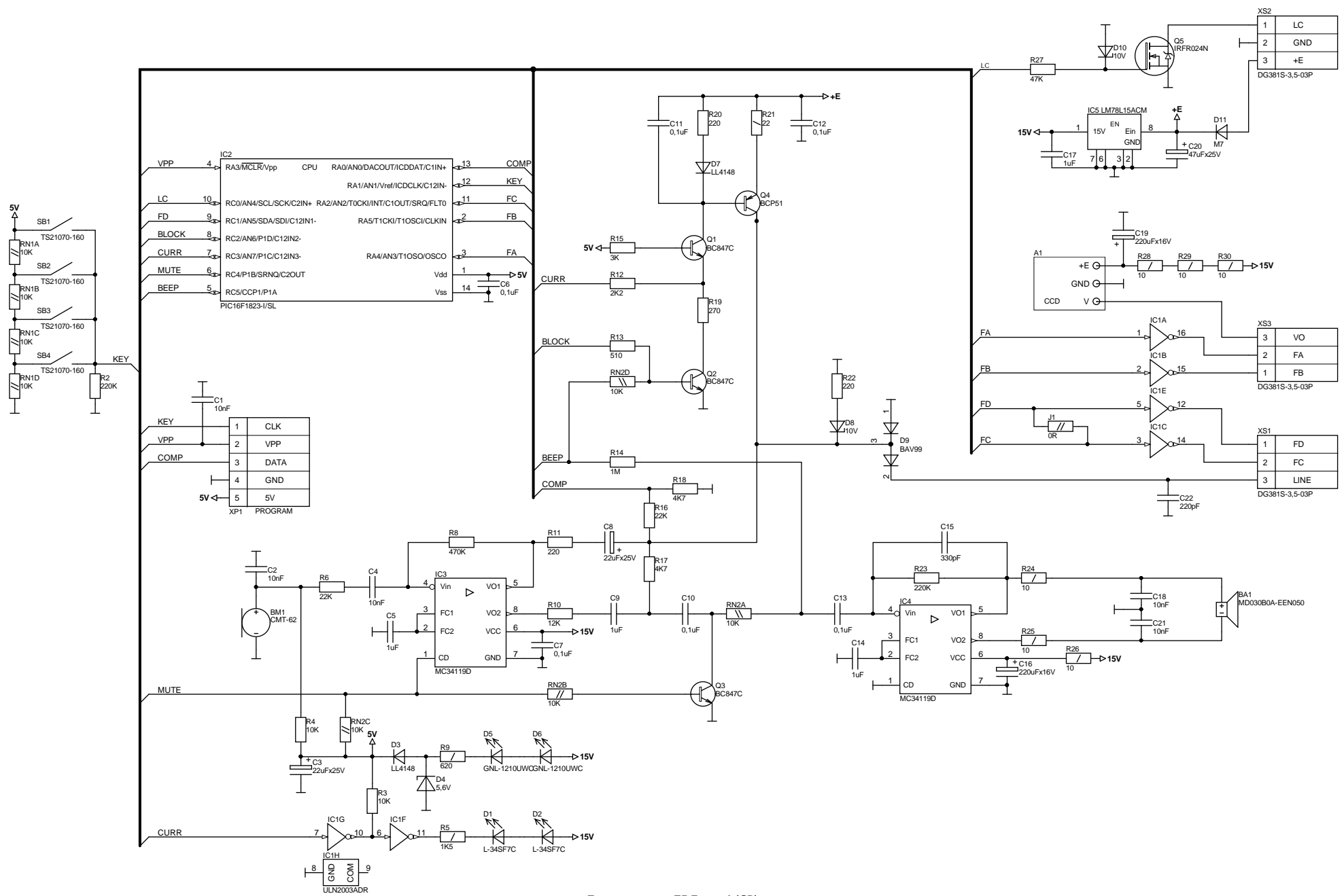
Блок вызова БВД-405А(СР)-2-4 Схема электрическая принципиальная
