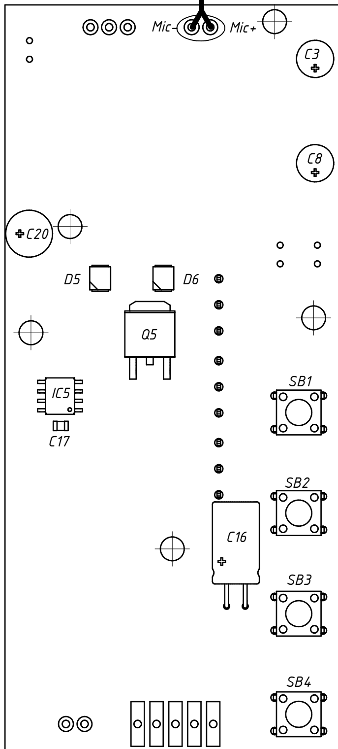
Плата БВД-405А-2, БВД-405А-4 Сборочный чертеж
