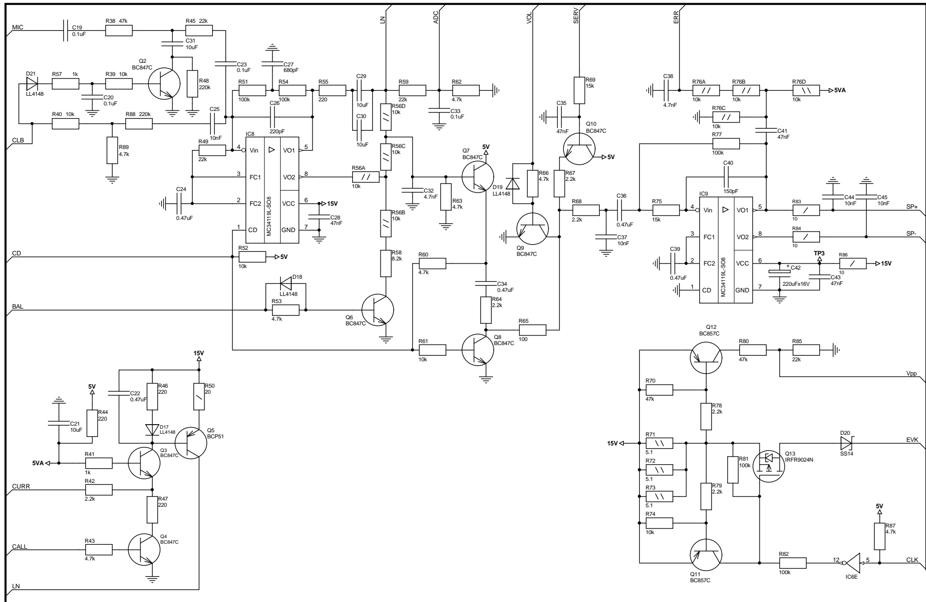
Блок управления БУД-430S(M) Схема электрическая принципиальная
