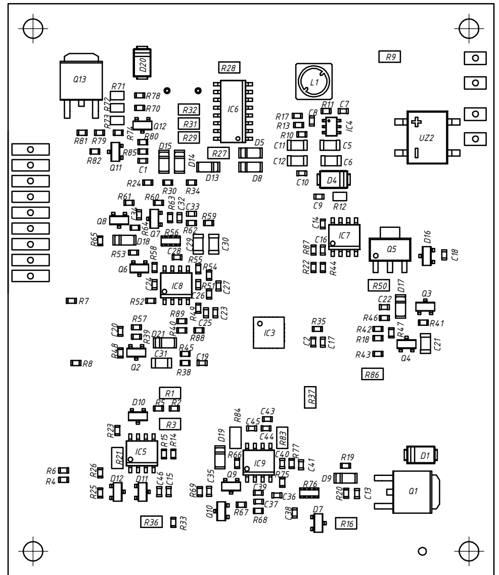
Плата БУД-430М Сборочный чертеж
