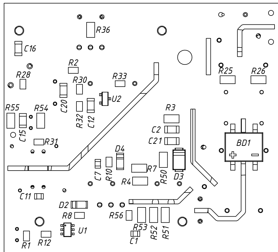
Плата модуля питания PM15VDC-20 Сборочный чертеж
