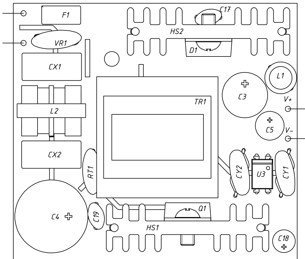
Плата модуля питания PM15VDC-20 Сборочный чертеж
