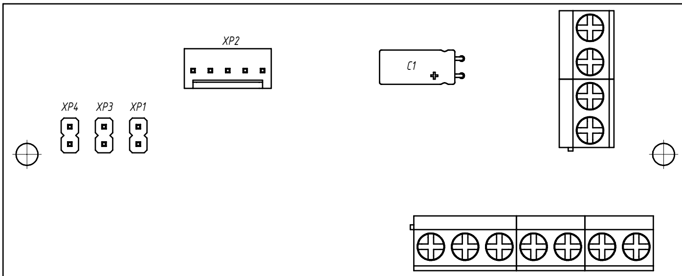
Плата БК-400 Сборочный чертеж
