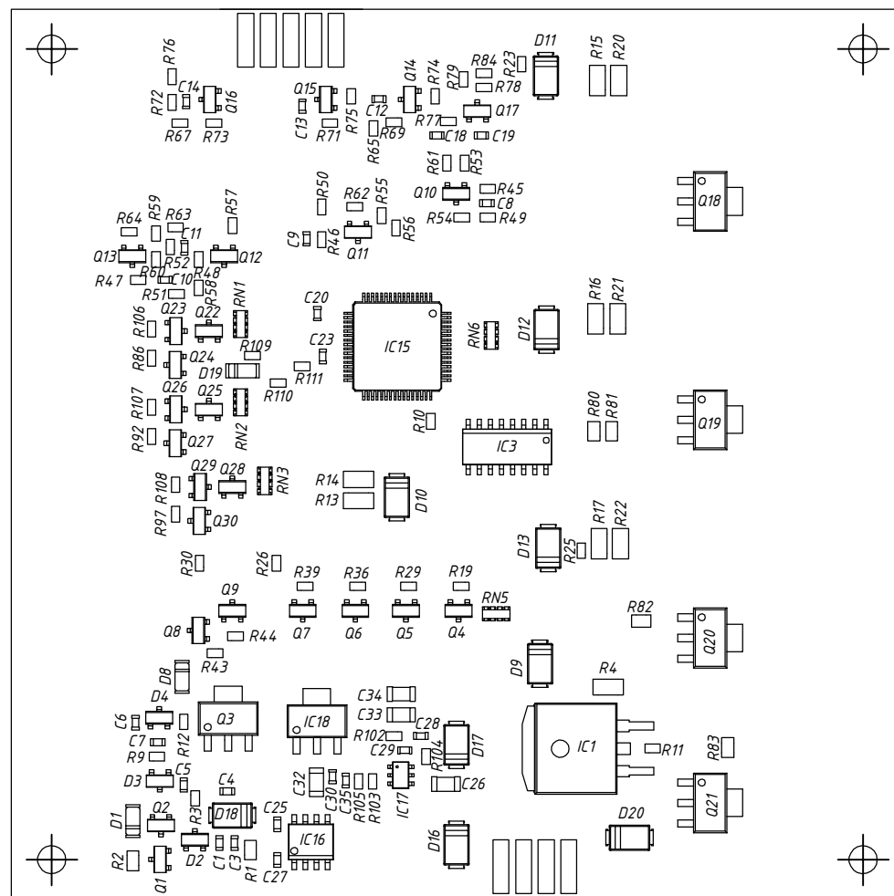
Плата БКМ-443 Сборочный чертёж
