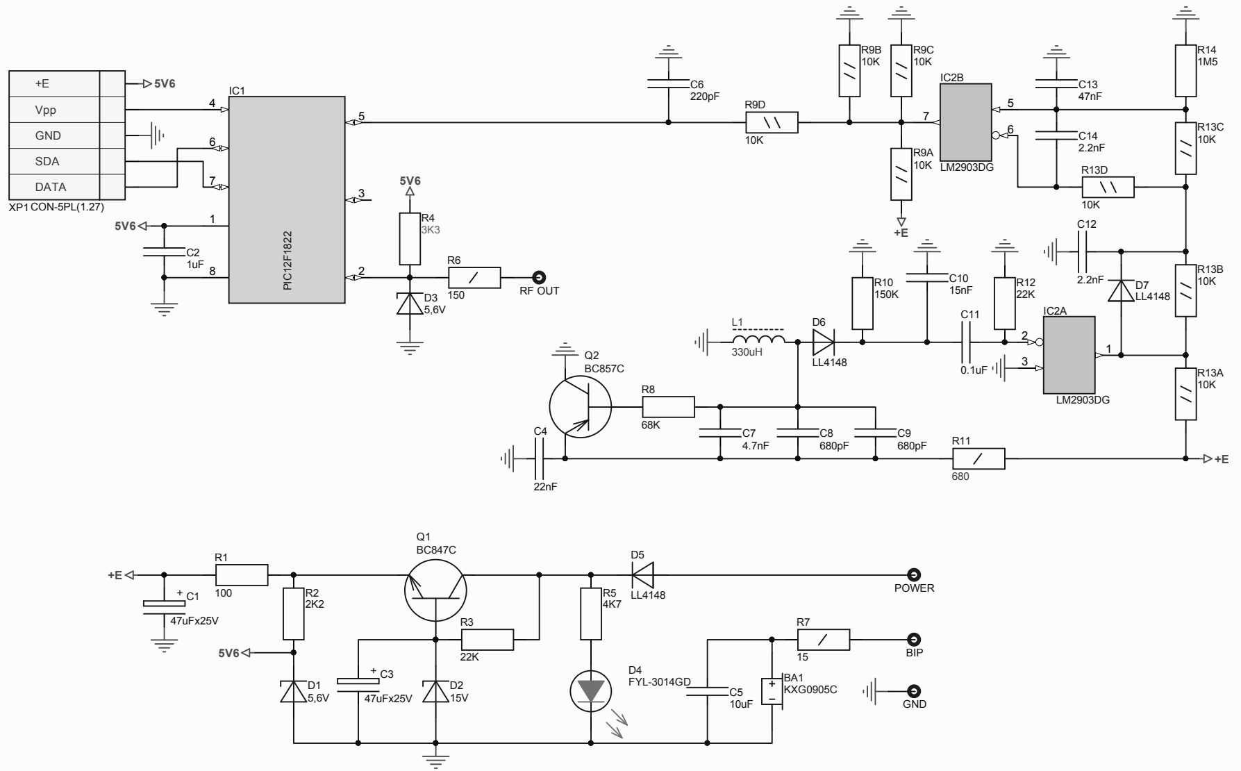
Считыватель RD-4R Схема элeтрическая принципиальная
