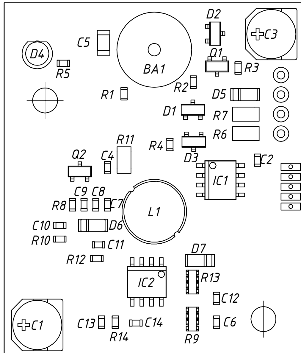
Плата считывателя RD-4R
