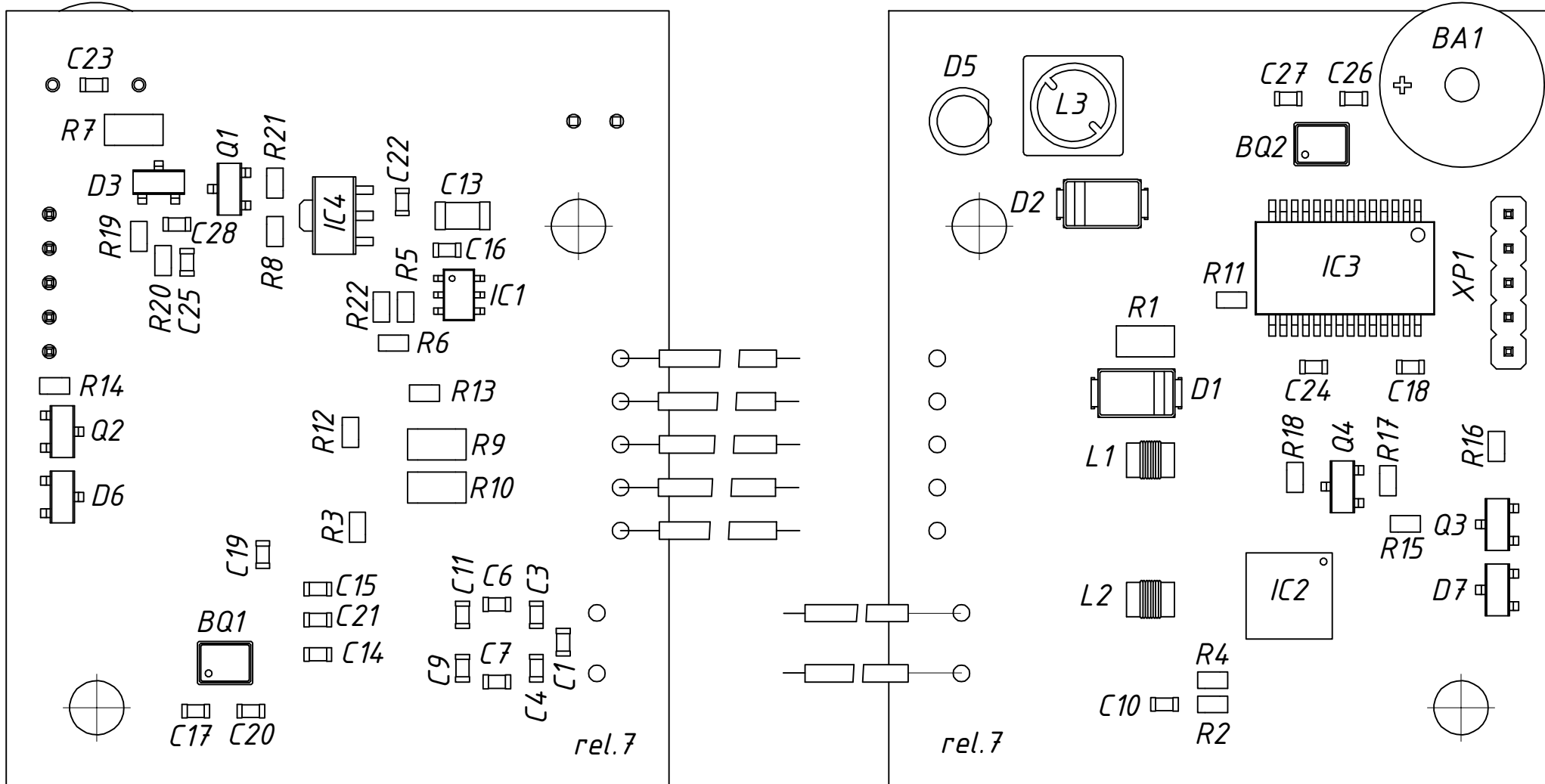
Плата считывателя RD-5F Сборочный чертеж
