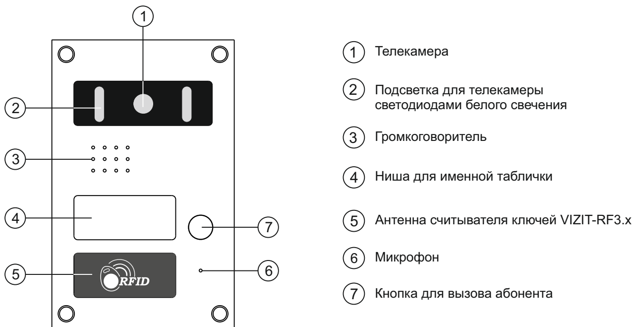
Внешний вид блока
