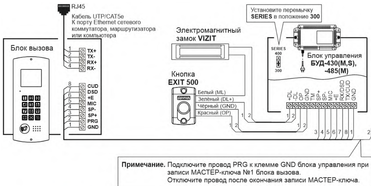
Рисунок 8.1 – Схема соединений блока вызова с блоком управления БУД-430(M,S), -480(S), -485(M,P), электромагнитным замком VIZIT-ML400 и кнопкой EXIT 1000
