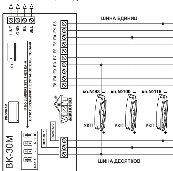
Блок коммутации БК-30М
